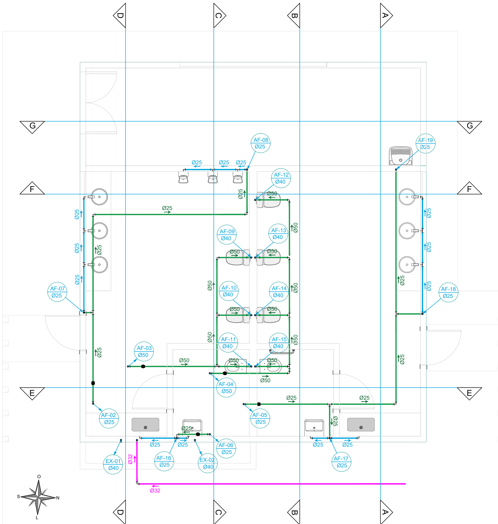
PLANTA BAIXA - REDE ÁGUA FRIA ESCALA 1:50
