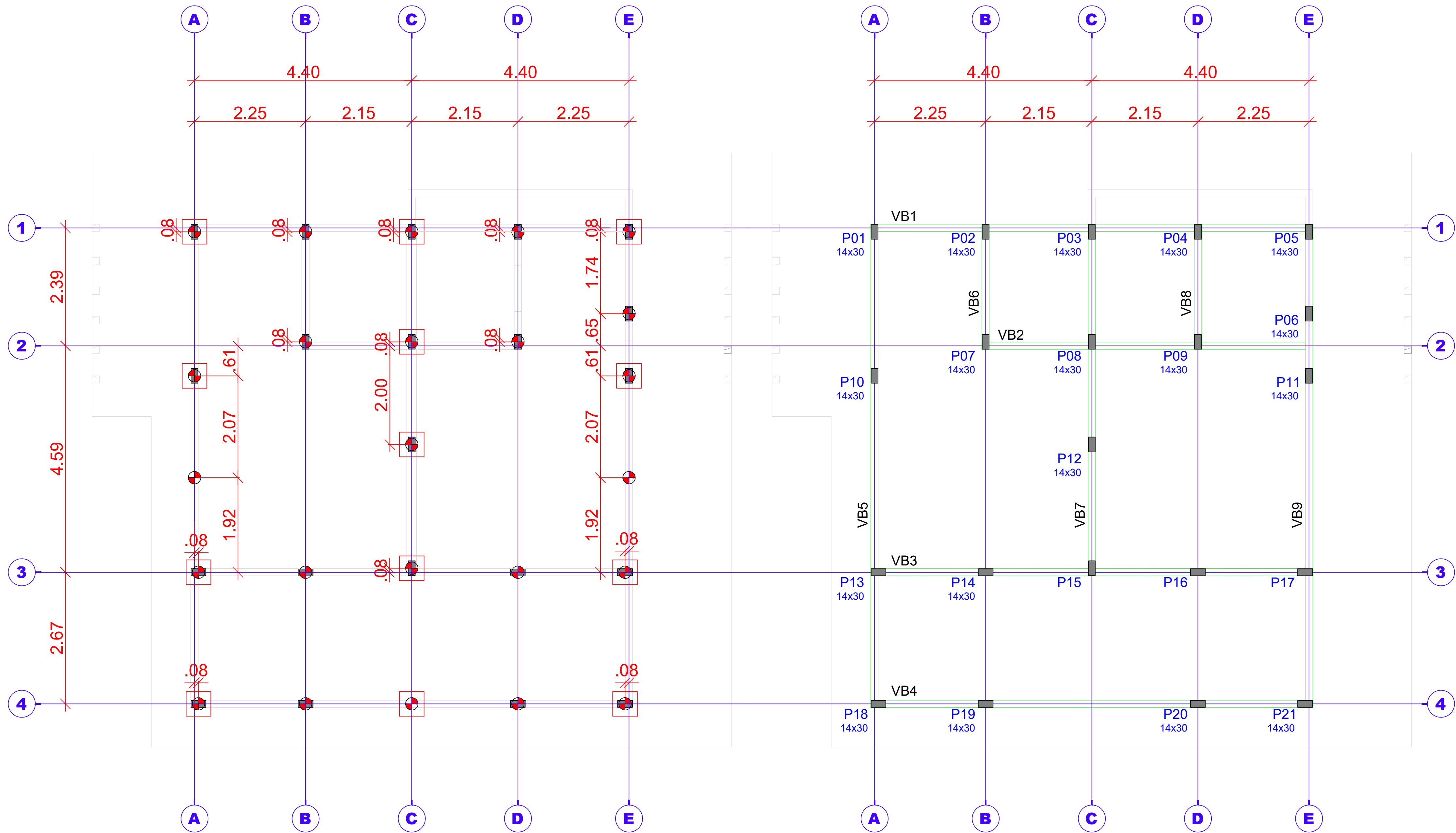
LOCAÇÃO DAS ESTACAS ESCALA 1:50
